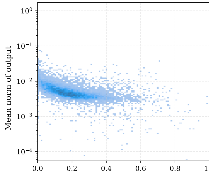
Layer 0
