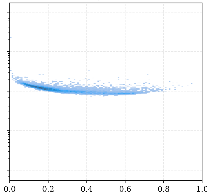
Layer 15
